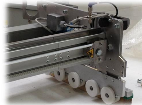
( Kit di allungamento )
