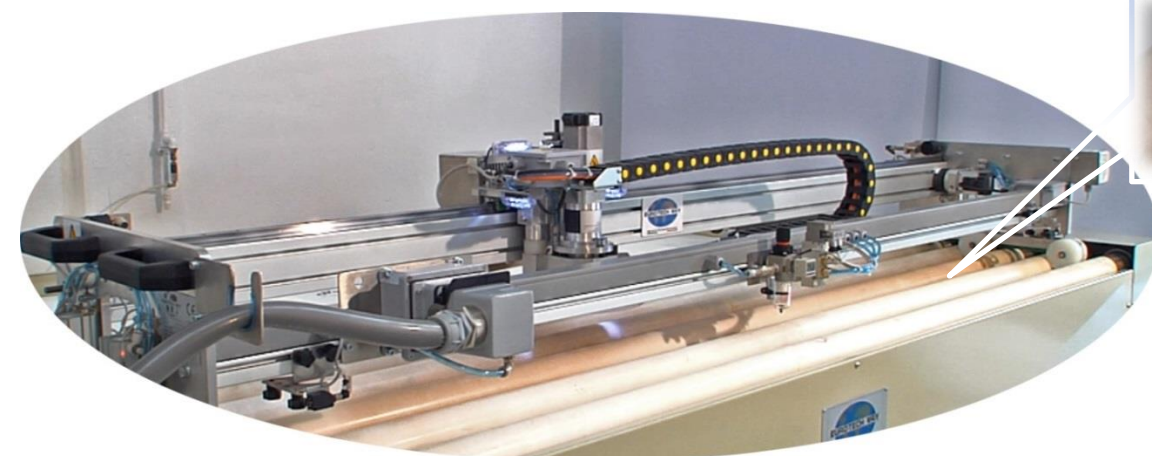
( Kit cambio passo per gestire passi diversi e diametro rulli diversi )
