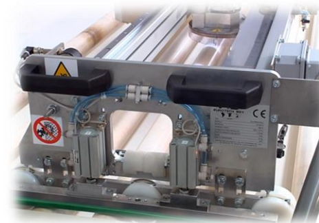
( Kit cambio passo per gestire passi diversi e diametro rulli diversi )
