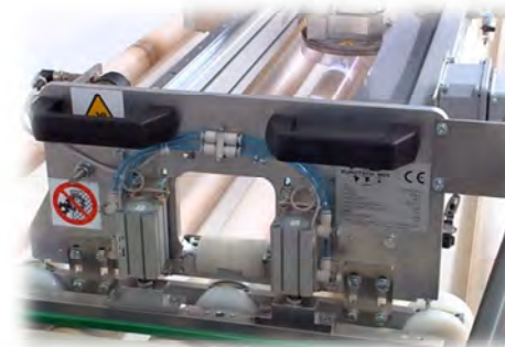
( cambio de paso de rodillos para gestionar diferente pasos y diferente diámetro rodillos
