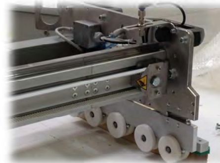
(dispositivo alargamiento )
