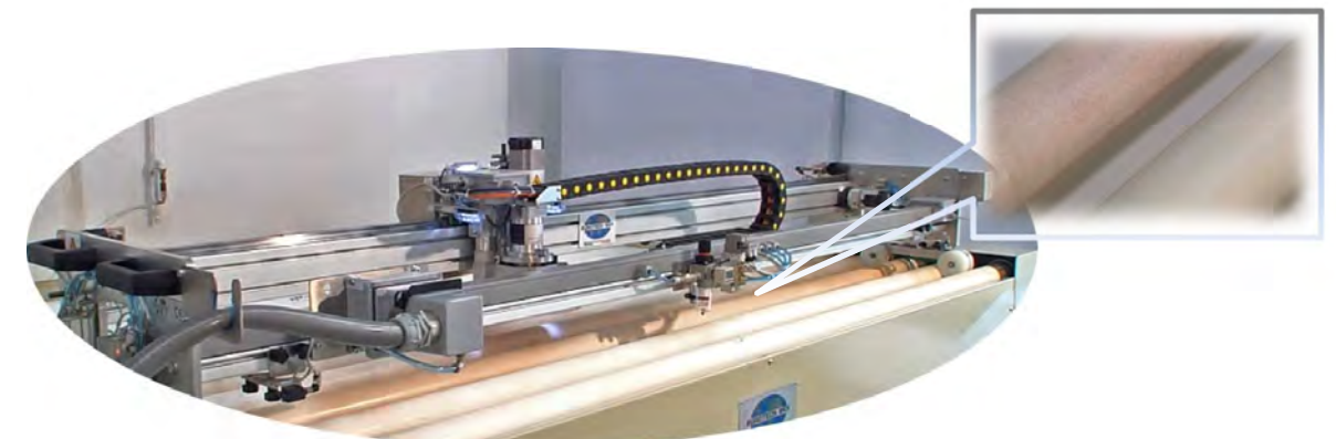
(dispositivo de cambio de paso de rodillos para gestionar diferente pasos y diferente diámetro rodillos)
